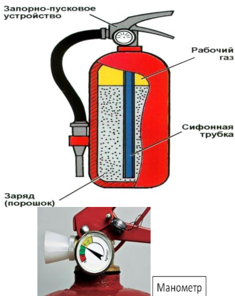
Рис. 31. Порошковые закачные огнетушители
