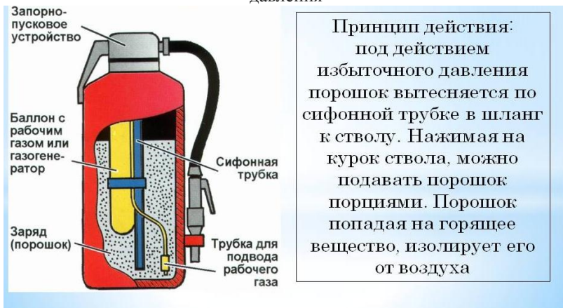
Рис. 28. Порошковые огнетушители со встроенным газовым источником давления
