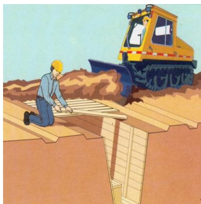
Рис. 11. Перекрытая щель
