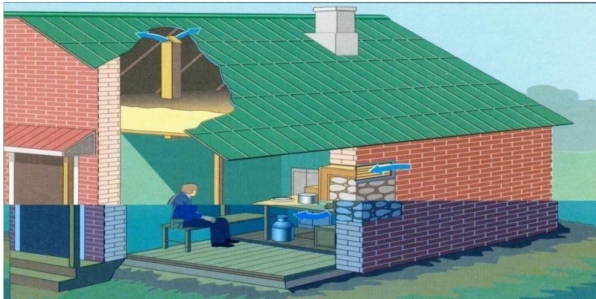
Рис. 8. Противорадиационное укрытие в индивидуальном жилом доме
