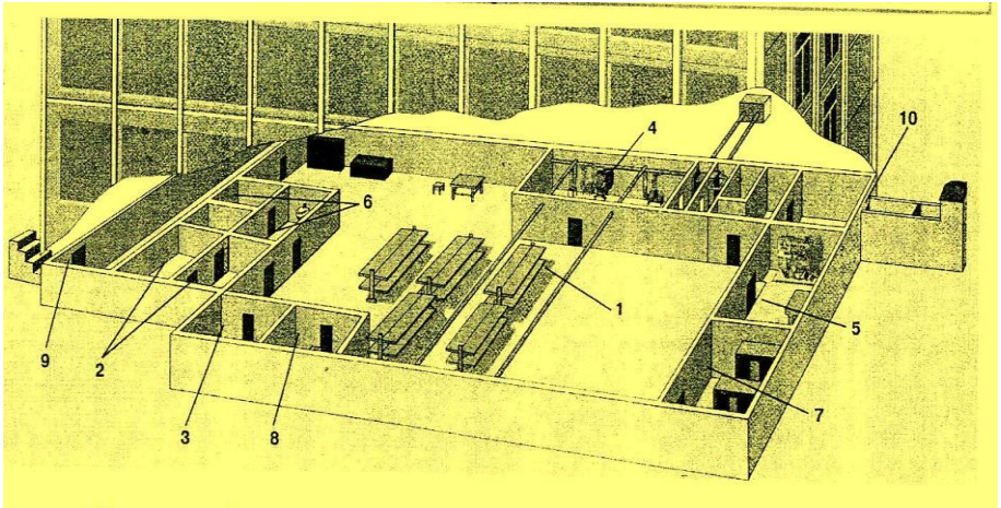
Рис. 6. Схема убежища
