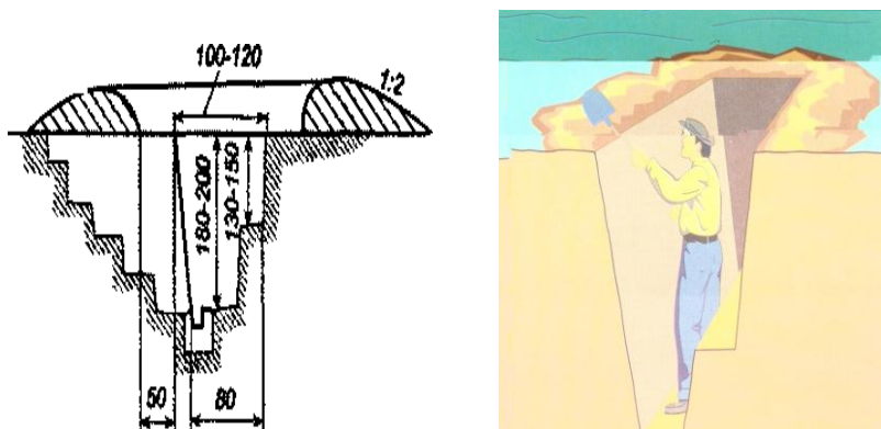
Рис. 10. Открытая щель
