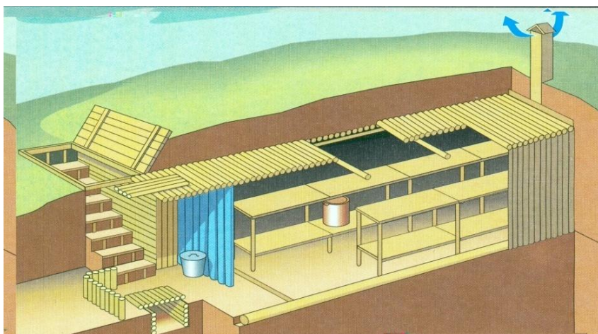
Рис. 9. Противорадиационное укрытие на открытой местности
